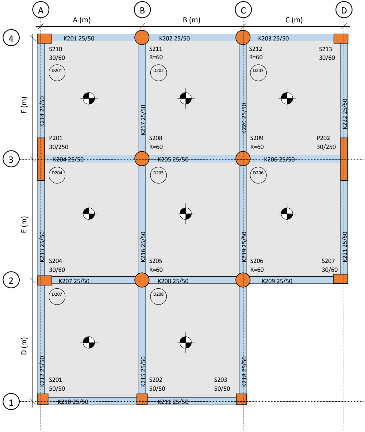
1. KAT ve 2. KAT TAVANI KALIP PLANI
